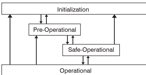
Abb. 75 EtherCAT State Machine
