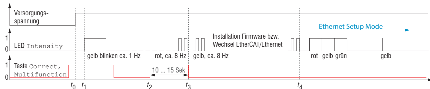
Abb. 132 Ablaufdiagramm für den Start eines IFx241x im Ethernet-Setup-Mode
