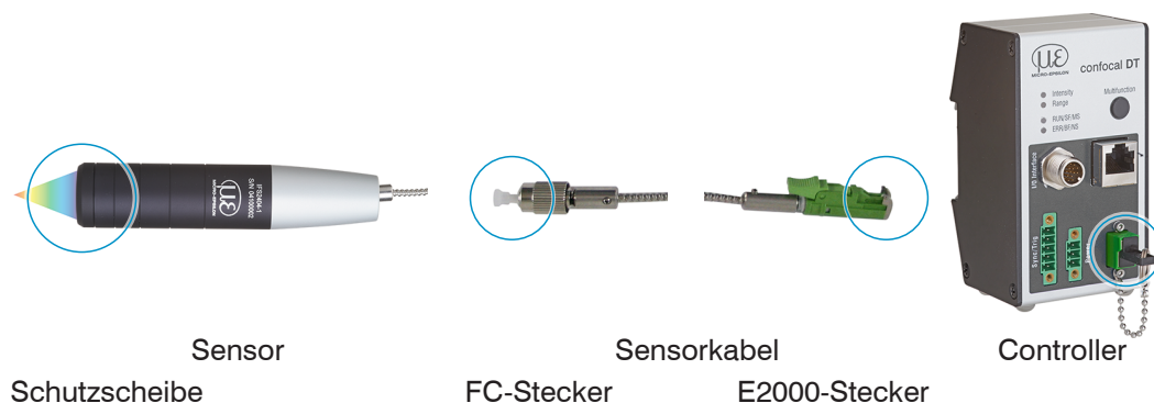
Abb. 126 Optische Grenzflächen eines konfokalen Messsystems
