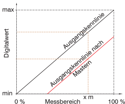
Abb. 62 Kennlinienverschiebung beim Mastern
