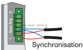
Abb. 26 Anschlüsse und Signalpegel interne Synchronisation
