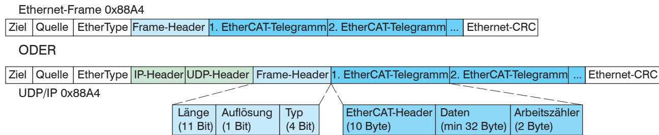
Abb. 74 Aufbau von EtherCAT-Frames
