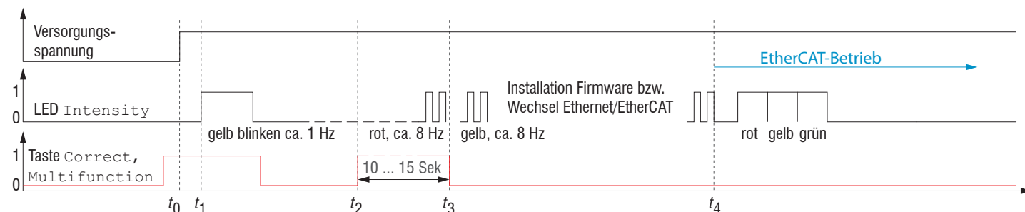
Abb. 133 Ablaufdiagramm für den Start eines IFx241x im EtherCAT-Betrieb
