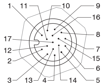
17-pol Sensorstecker, Pinseite
