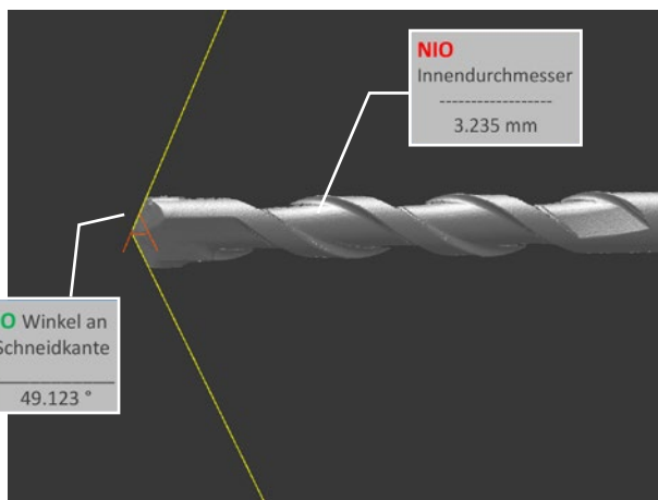
Messung des Spitzenwinkels der Hauptschneide eines Bohrkopfes sowie Messung des Innendurchmessers
