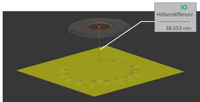
Höhendifferenzmessung der Bohrung in einem Zahnrad
