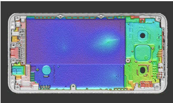
Erkennung von Oberflächendefekten auf einer Smartphone-Schale
