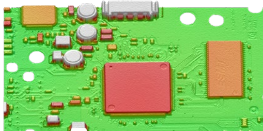
Vollständigkeitsprüfung elektronischer Bauteile auf bestückter Leiterplatte
