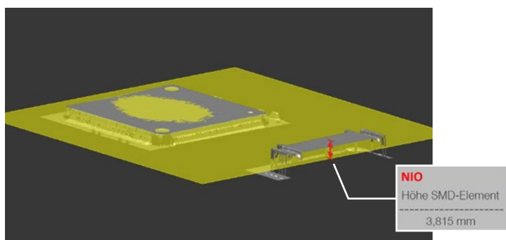
Überwachung von Abstand und Planparallelität der bestückten Elemente zueinander und zur Grundfläche (z.B. bei Tombstone-Effekt)
