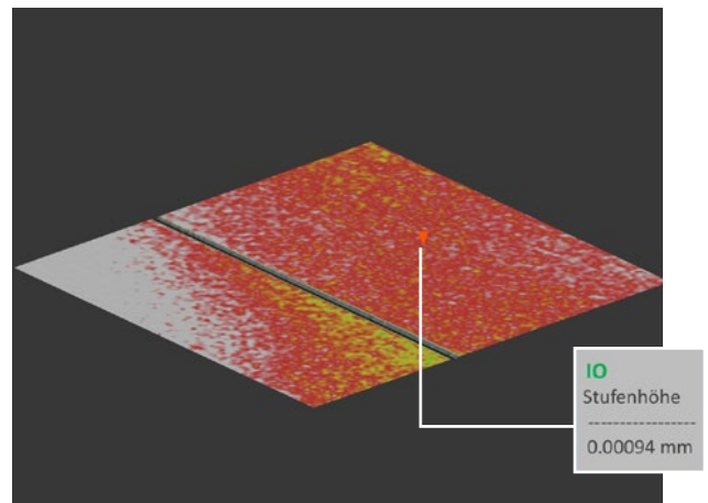
Zuverlässige und hochpräzise Messung einer 1 \mu\text{m} hohen Stufe Darstellung einer Höhendifferenz.
